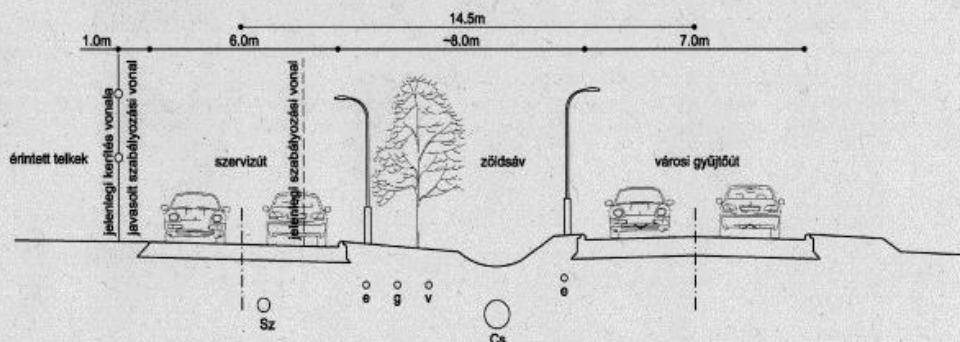
Javasolt útépitési mintakeresztmetszévény közműelhelyezéssel
